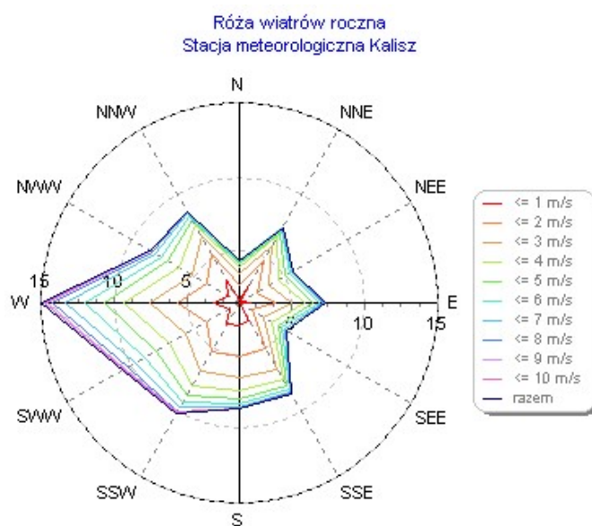
Rycina 4. Róża wiatrów - stacja meteorologiczna Kalisz
